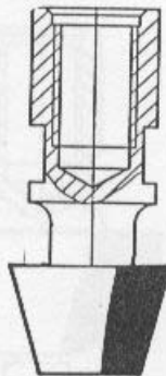
Kantenfräser, konisch wahlweise mit 15° und 45°
