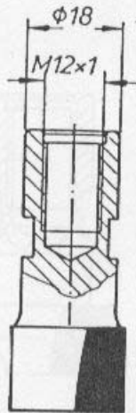
Kantenfräser, zylindrisch
