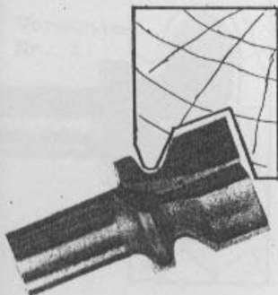
Fräsvorschlag Nr. 3 Schrägfräsung (durch Unterlegen mittels Keil)
