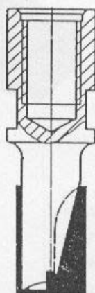
Nutfräser M 12×1
