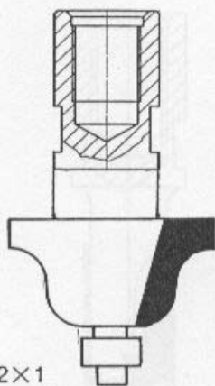
Bestell-Nr. 311 M 12×1
