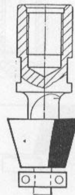
Kantenfräser, konisch wahlweise mit 15° und 45°
