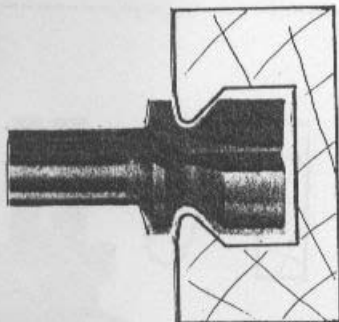
Fräsvorschlag Nr. 3 Schrägfräsung (durch Unterlegen mittels Keil)
