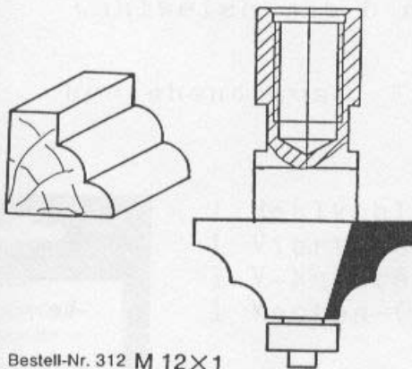
Bestell-Nr. 312 M 12×1
